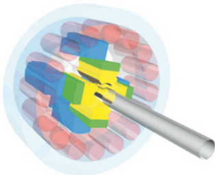
Das Rundkneten (Hämmern) ist ein inkrementelles Umformverfahren für die Reduzierung des Querschnittes von Stäben, Rohren und Drähten.
